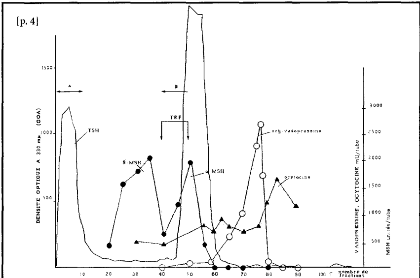
Fig. 1. Fractionnement d'un extrait acétique d'hypothalamus de mouton sur colonne de « Sephadex G-25 ». 4,9 g de l'extrait sont filtrés sur une colonne de 5,5 x 90 cm équilibrée avec le tampon acétate de pyridinium 0,1 M, pH 5. Débit de la colonne : 50 à 60 ml/h. Volume des fractions : 20 ml. Des prises de 0,3 ml de chaque fraction sont utilisées pour le dosage colorimétrique au biuret à 330 nm (J. GOA, Scand. J. Clin. Lab. Inv. , 5 1953, p. 218; A. V. SCHALLY et R. GUILLEMIN, Texas Reports Biol. Med. , 18, 1960, p. 133). Les fractions sont réunies deux par deux et lyophilisées. Pour le dosage de l'activité TRF, on utilise l'équivalent de 2,0 ml de l'effluent original, par animal.
